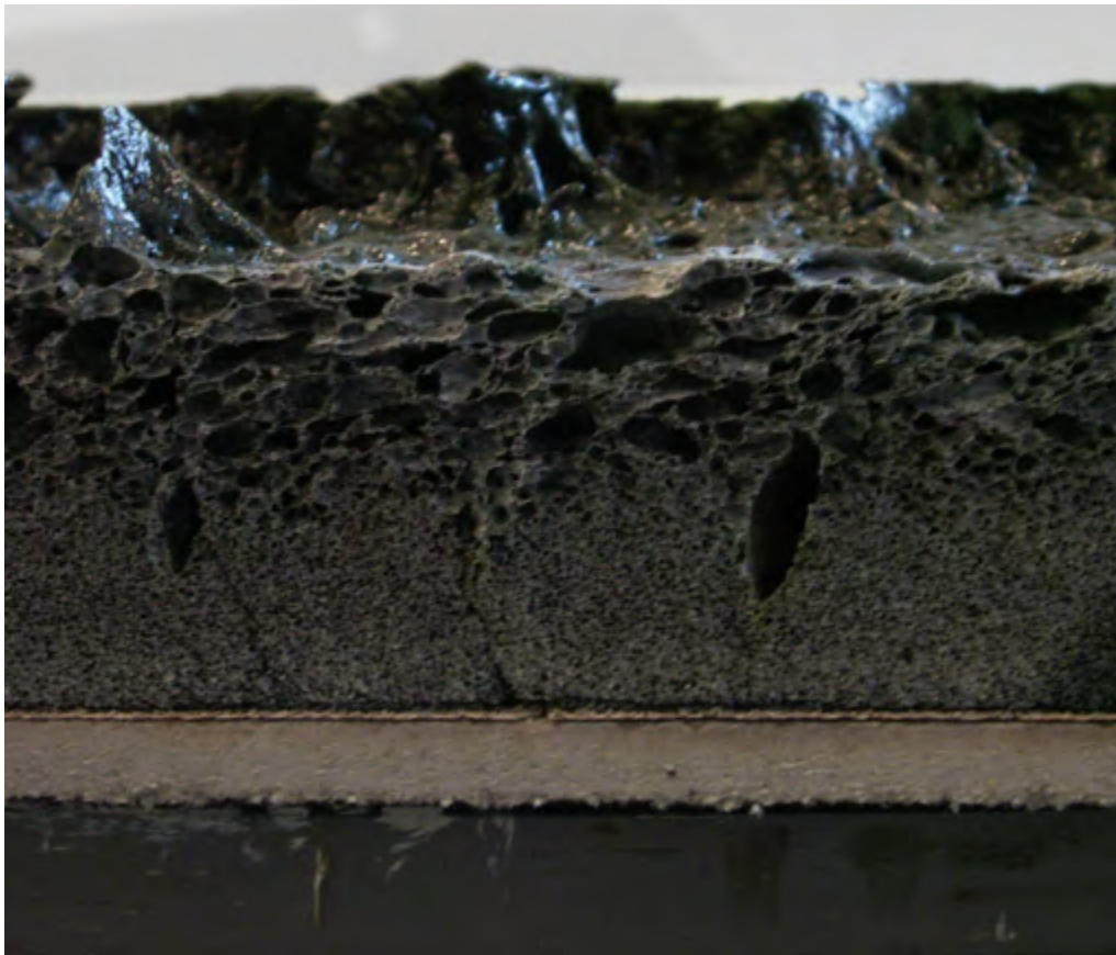
Testcertificaat van de Materialprüfanstalt Braunschweig (Duitsland). FOAMGLAS® mag worden omschreven als een product met een smeltpunt van minstens 1.000 °C.
