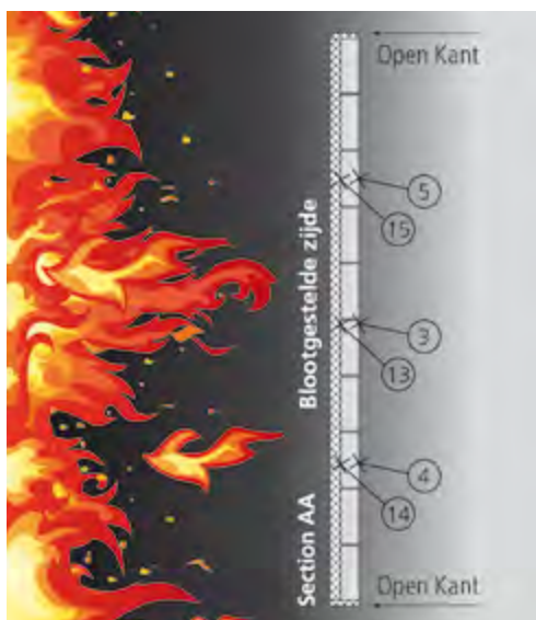
Opbouw testwand voor brandweerstandsproeven.
